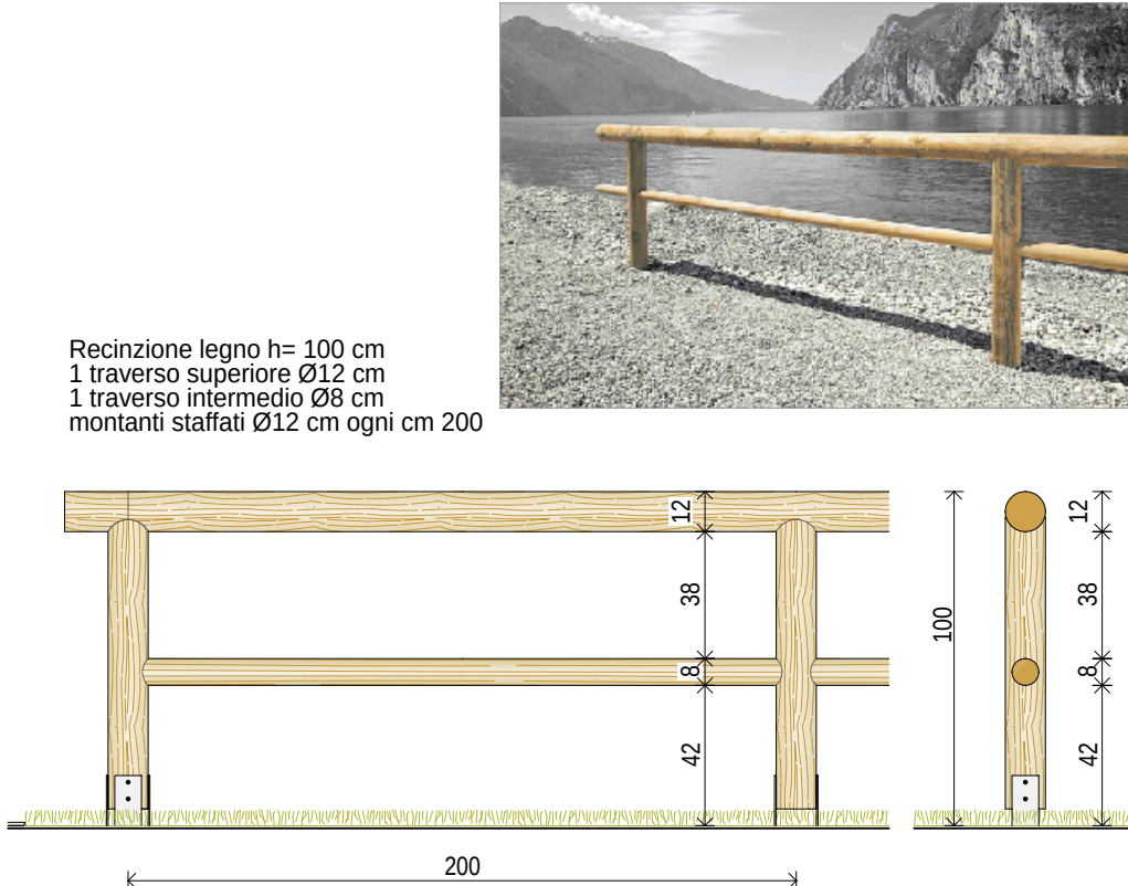
Recinzione in legno
