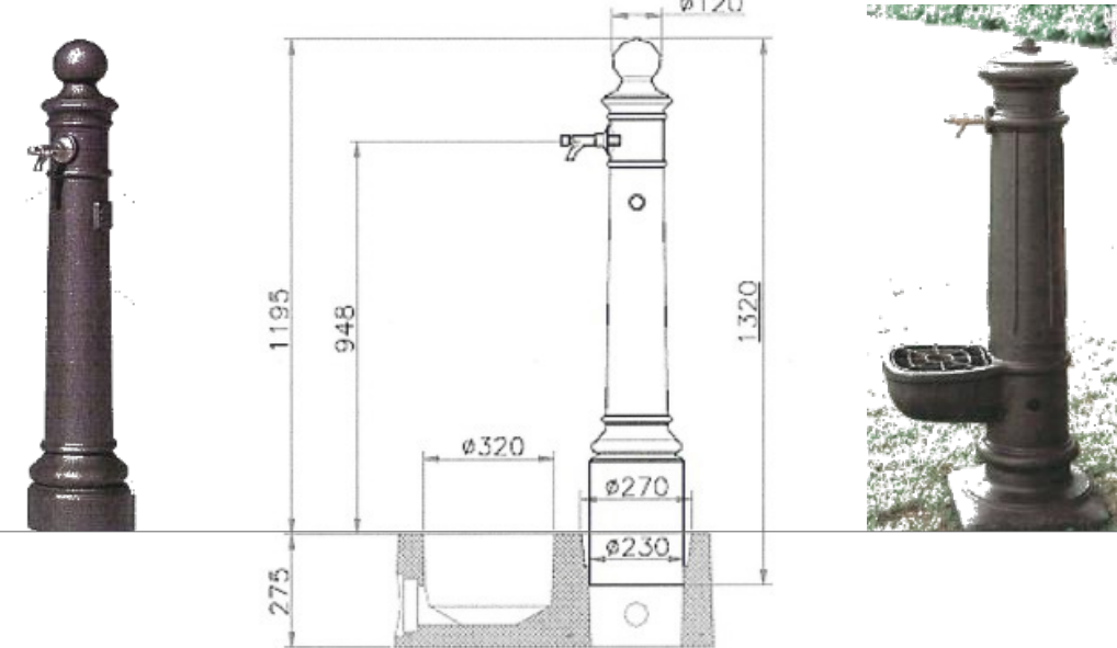
Fontana senza basamento e fontana con tazza (area cani)
