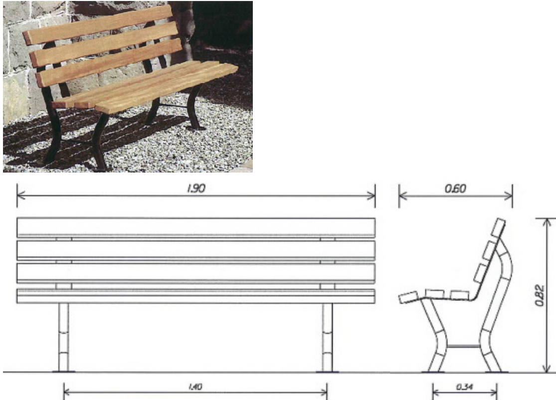
Panchina in legno 6 listoni
