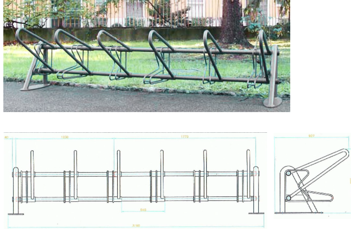
Portabicicletta modello "Verona" 6 posti - stalli ortogonali
